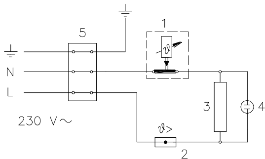
Schema für den Anschluss an die Elektroleitung
